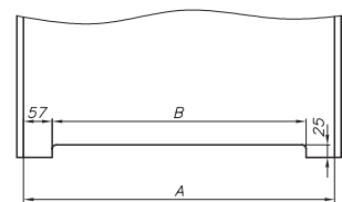
skrzydło FIORD / IMPULS z podcięciem wentylacyjnym
